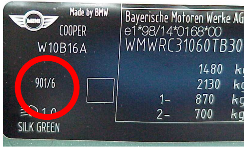
VIN PLATE MINI PAINTCODE = 901
